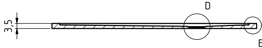
Sección C-C
