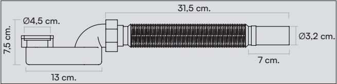
(sifón incluido) • (siphon included) • (siphon inclus) (sifone incluso) • (Siphon enthalten)
