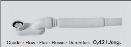
Caudal • Flow • Flux • Flusso • Durchfluss 0,42 l./seg.
