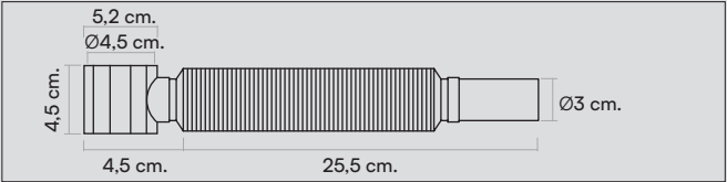
(sifón no incluido) • (siphon not included) • (siphon non inclus) (sifone non incluso) • (Siphon nicht enthalten)
