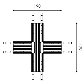
X-JOINT
