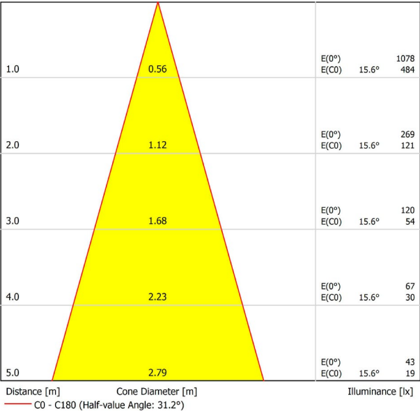
KEGELDIAGRAMM
