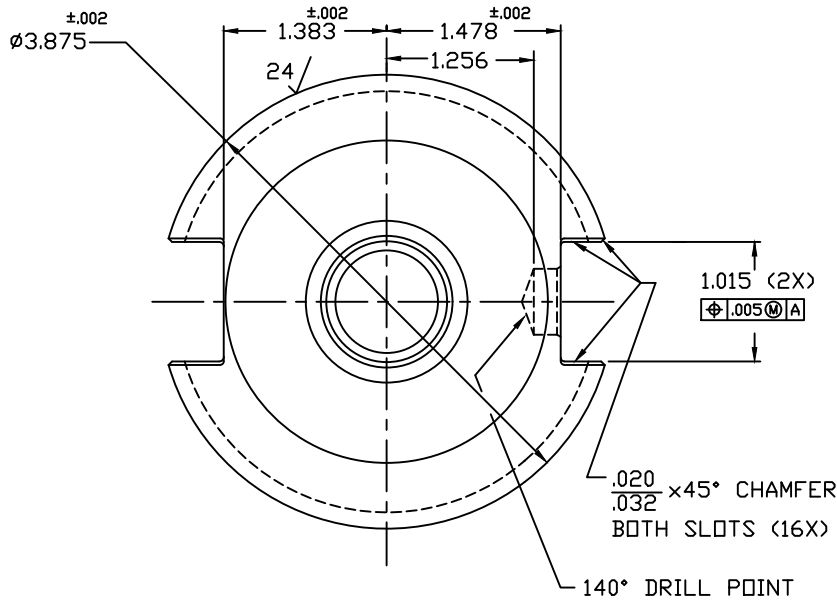
VIEW A-A
