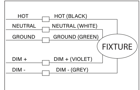
WIRING DIAGRAM (0-10)
